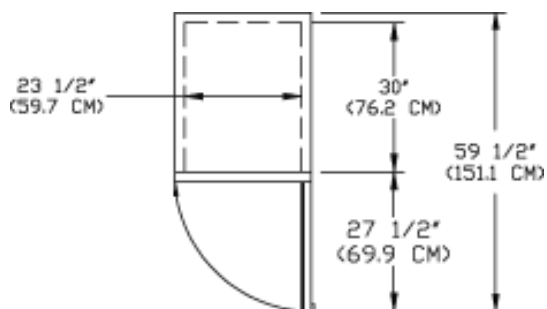
TOP - NSZF241WMW/_M
