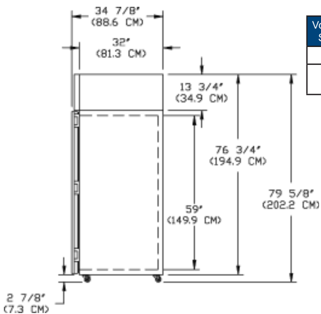
SIDE - NSZF241WMW/_M
